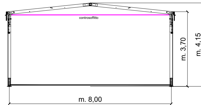
SEZIONE CENTRALE
