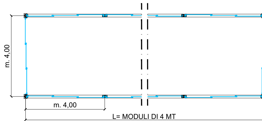
PLANIMETRIA
