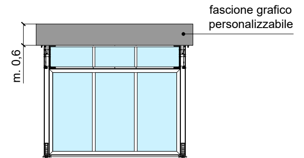
PROSPETTO FRONTALE
