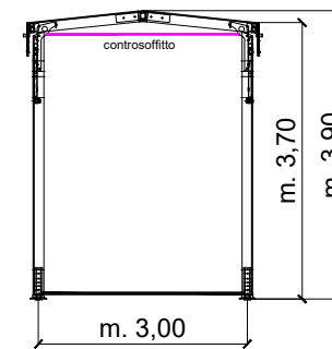
SEZIONE CENTRALE
