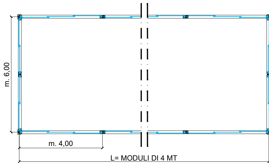
PLANIMETRIA
