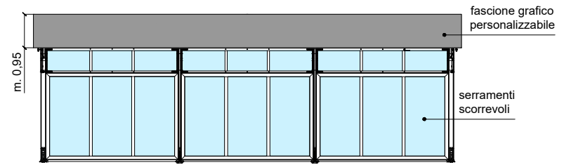
PROSPETTO FRONTALE
