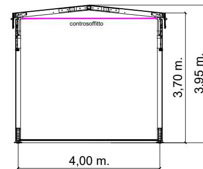
SEZIONE CENTRALE
