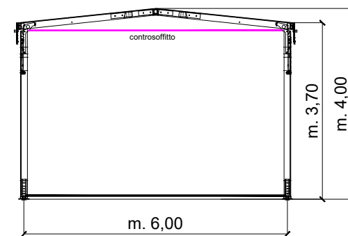
SEZIONE CENTRALE
