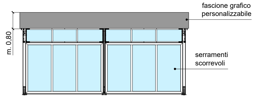
PROSPETTO FRONTALE
