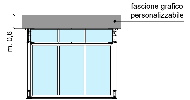
PROSPETTO FRONTALE
