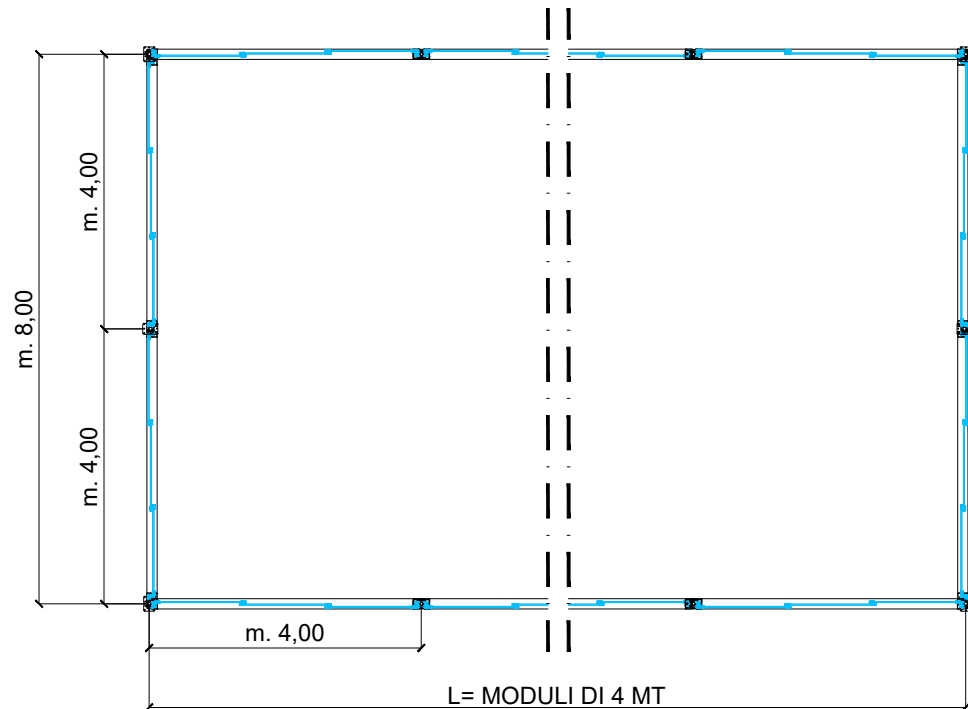
PLANIMETRIA
