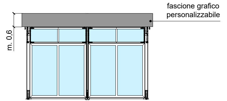
PROSPETTO FRONTALE
