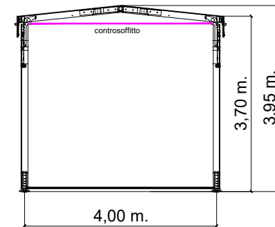
SEZIONE CENTRALE
