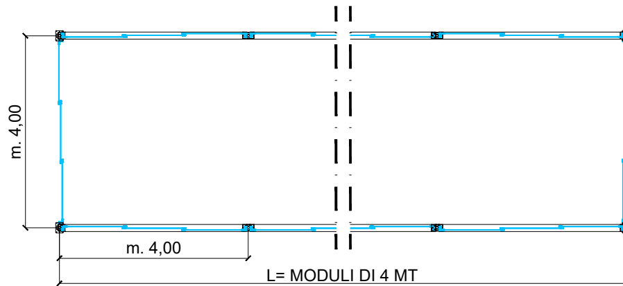
PLANIMETRIA
