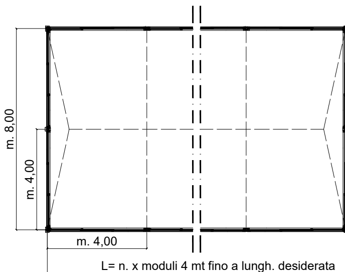
PLANIMETRIA
