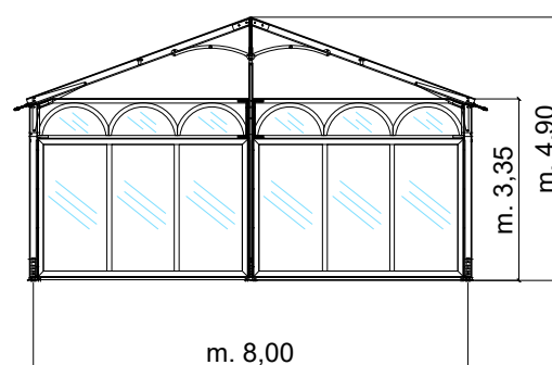
PROSPETTO FRONTALE
