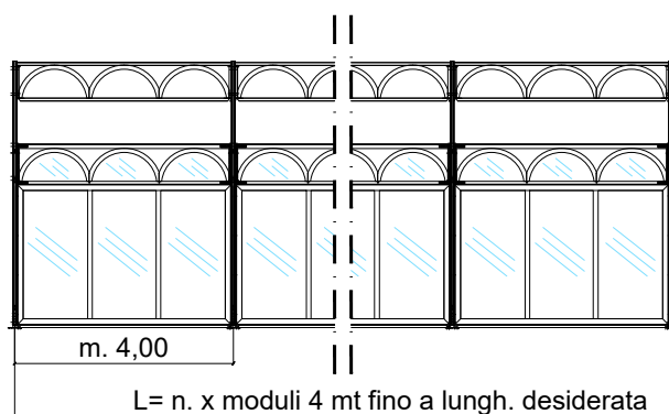
PROSPETTO LATERALE
