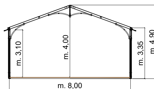
SEZIONE CENTRALE
