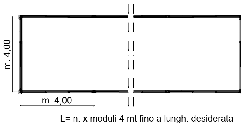
PLANIMETRIA
