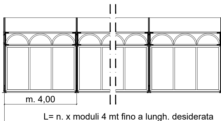
PROSPETTO LATERALE
