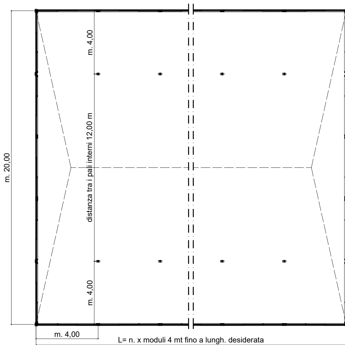
PLANIMETRIA
