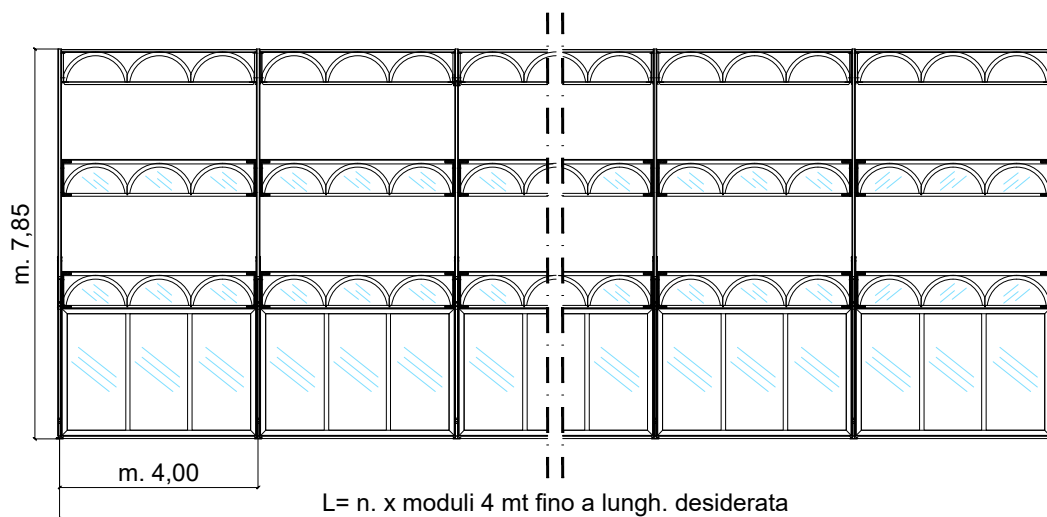
PROSPETTO LATERALE
