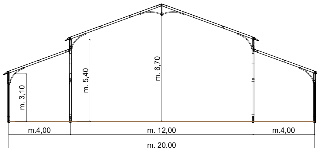
SEZIONE CENTRALE
