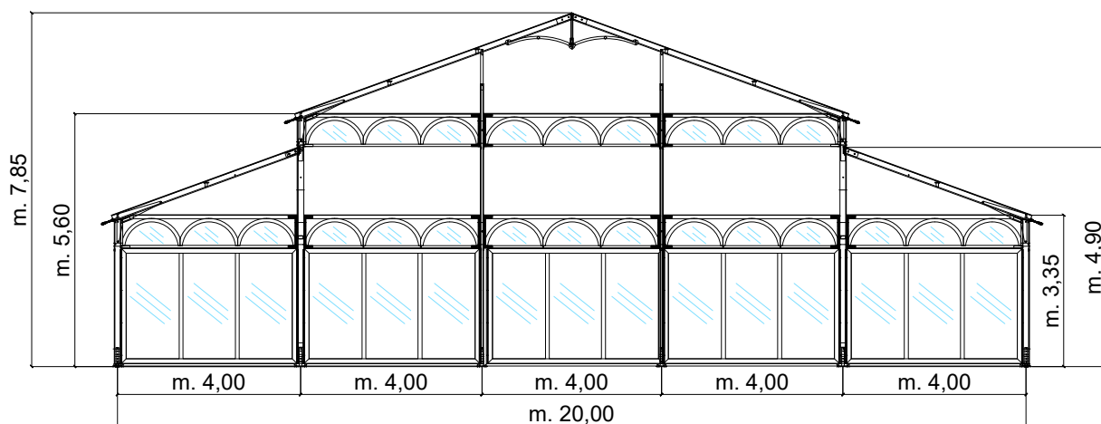
PROSPETTO FRONTALE
