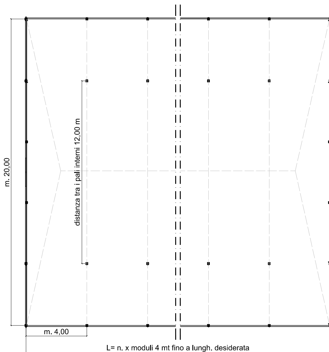
PLANIMETRIA
