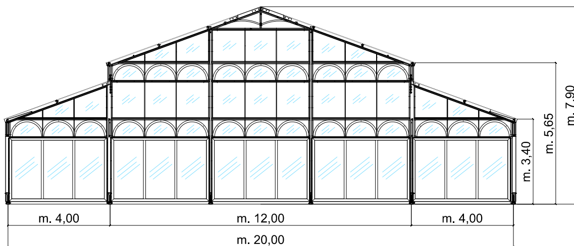
PROSPETTO FRONTALE
