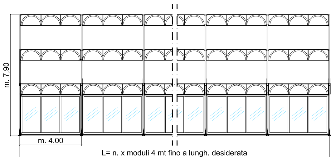
PROSPETTO LATERALE
