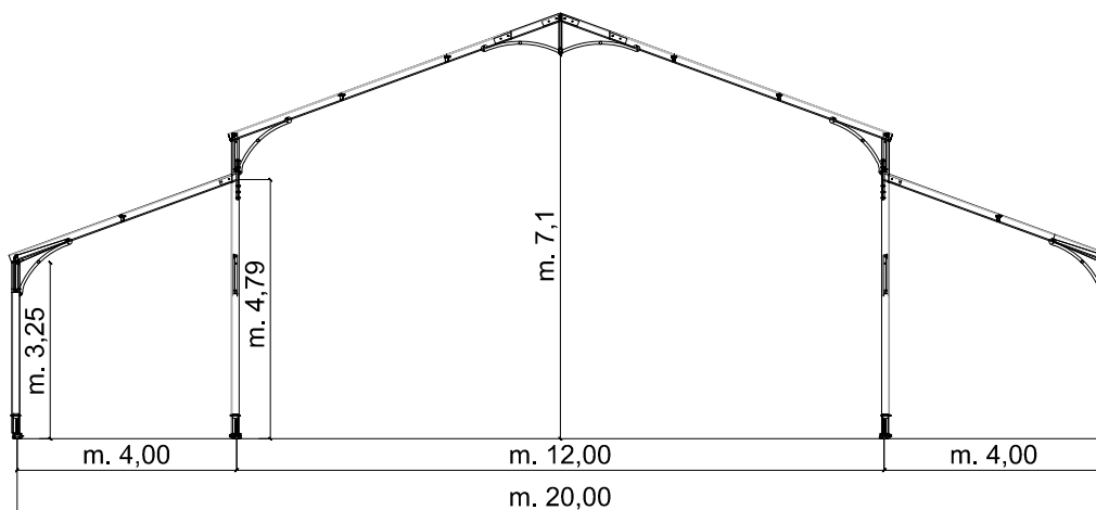
SEZIONE CENTRALE
