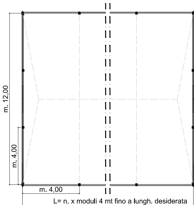
PLANIMETRIA
