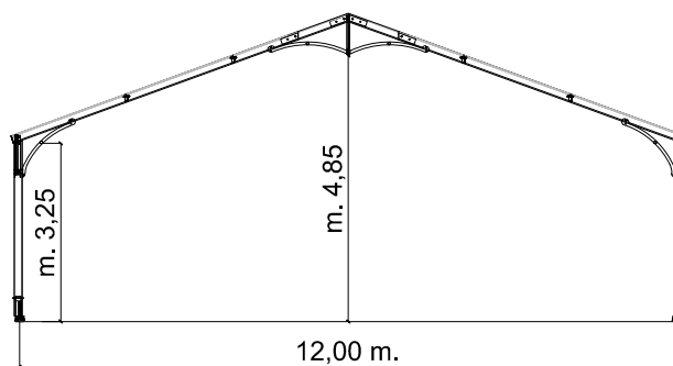
SEZIONE CENTRALE
