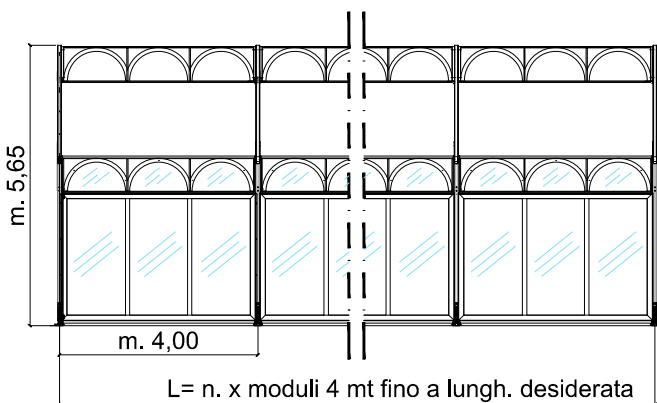
PROSPETTO LATERALE
