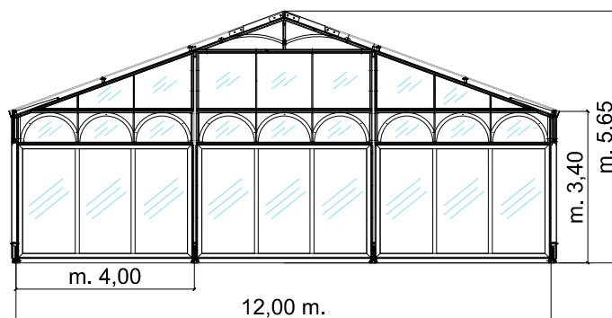
PROSPETTO FRONTALE
