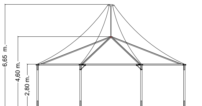
PROSPETTO
