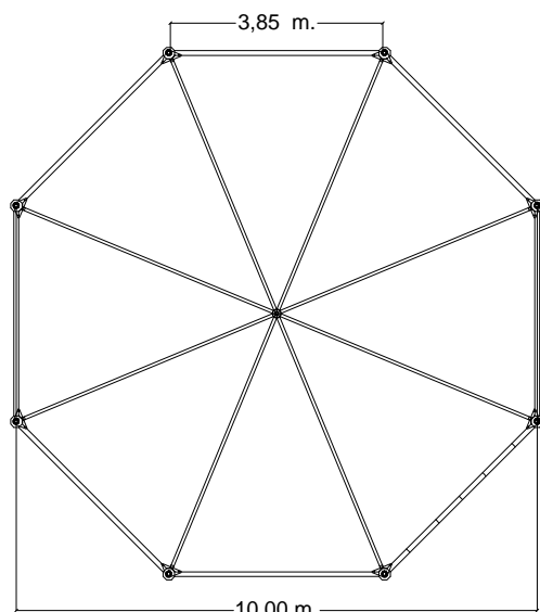
PLANIMETRIA
