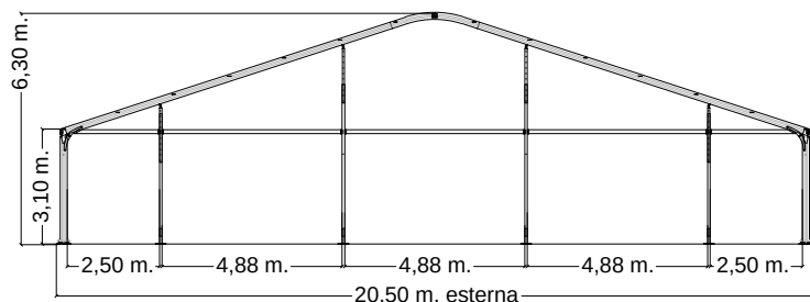
PROSPETTO FRONTALE
