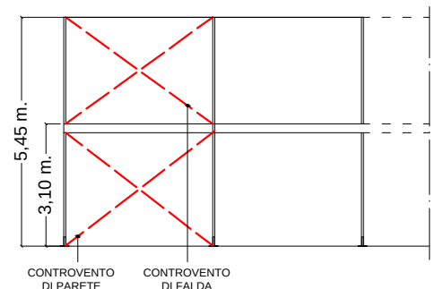
PROSPETTO LATERALE
