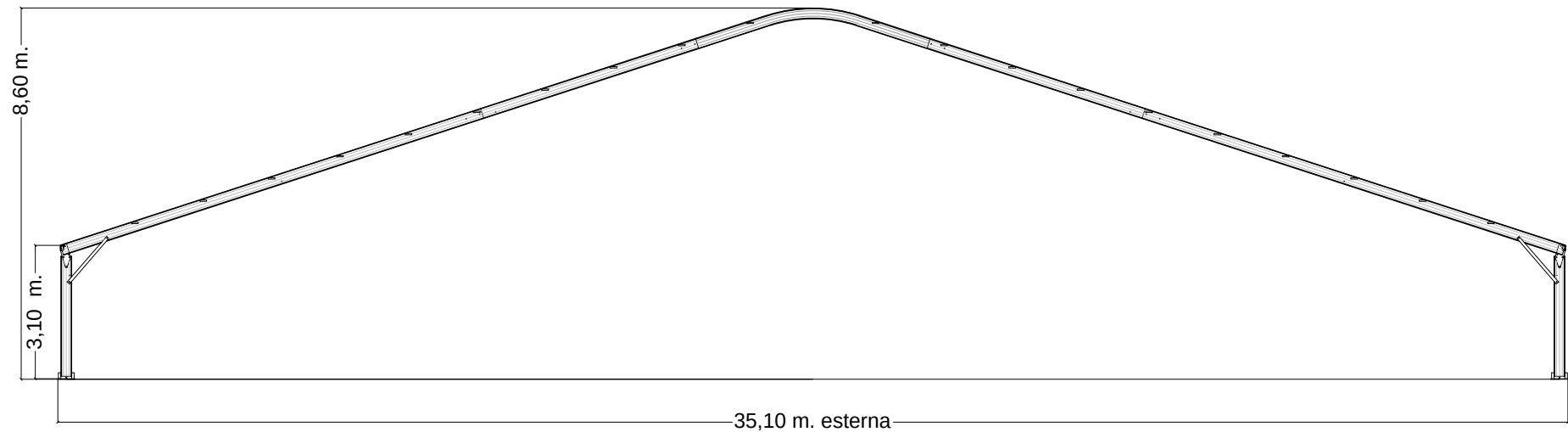
SEZIONE CENTRALE
