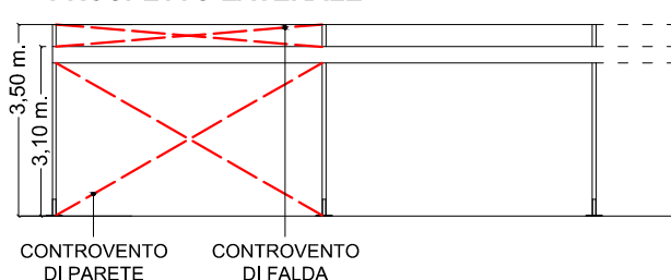
PROSPETTO LATERALE
