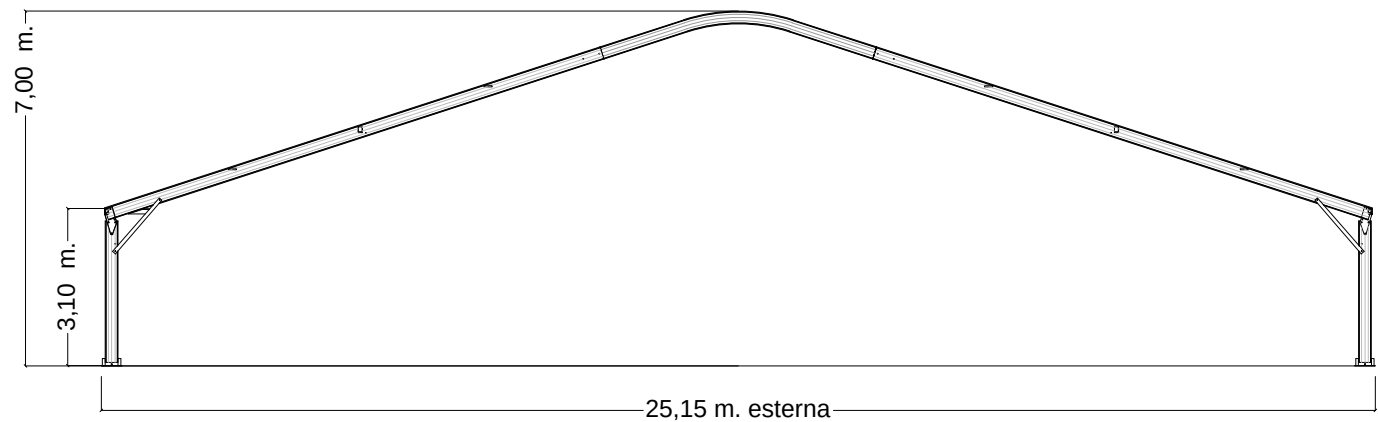
SEZIONE CENTRALE
