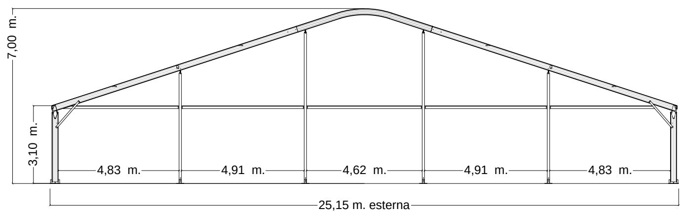
PROSPETTO FRONTALE
