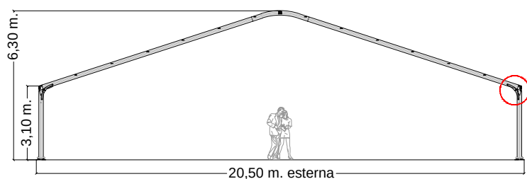
SEZIONE CENTRALE
