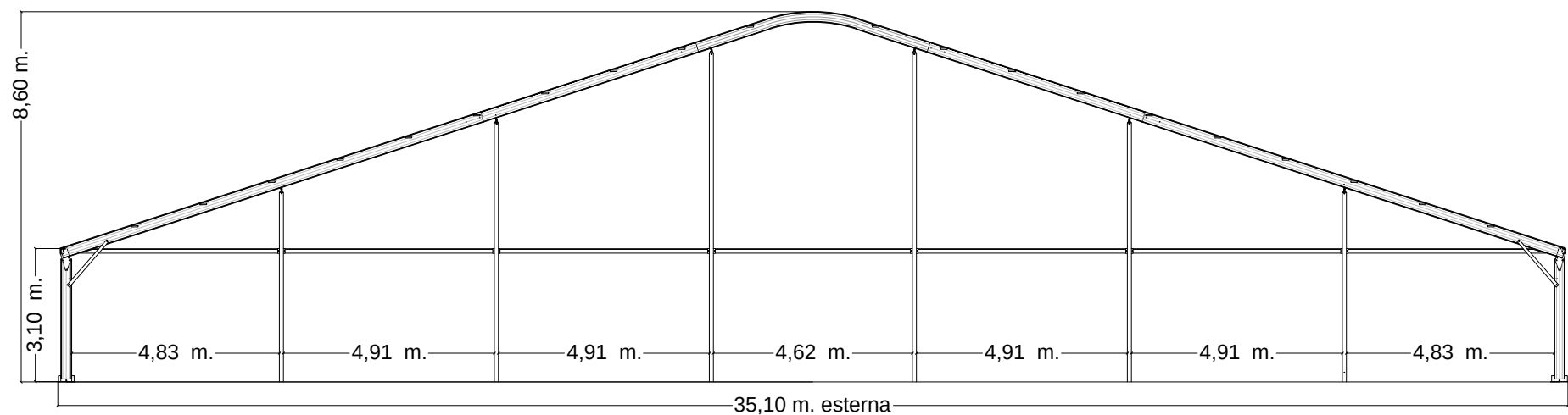
SEZIONE CENTRALE
