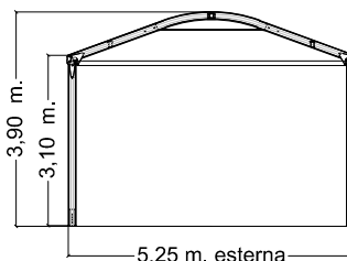
PROSPETTO FRONTALE
