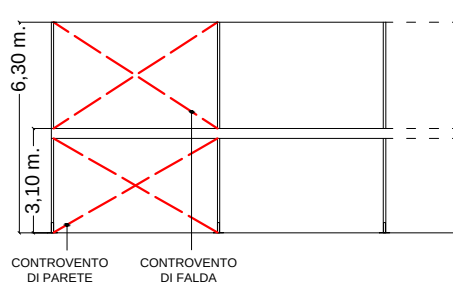
PROSPETTO LATERALE
