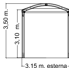
PROSPETTO FRONTALE
