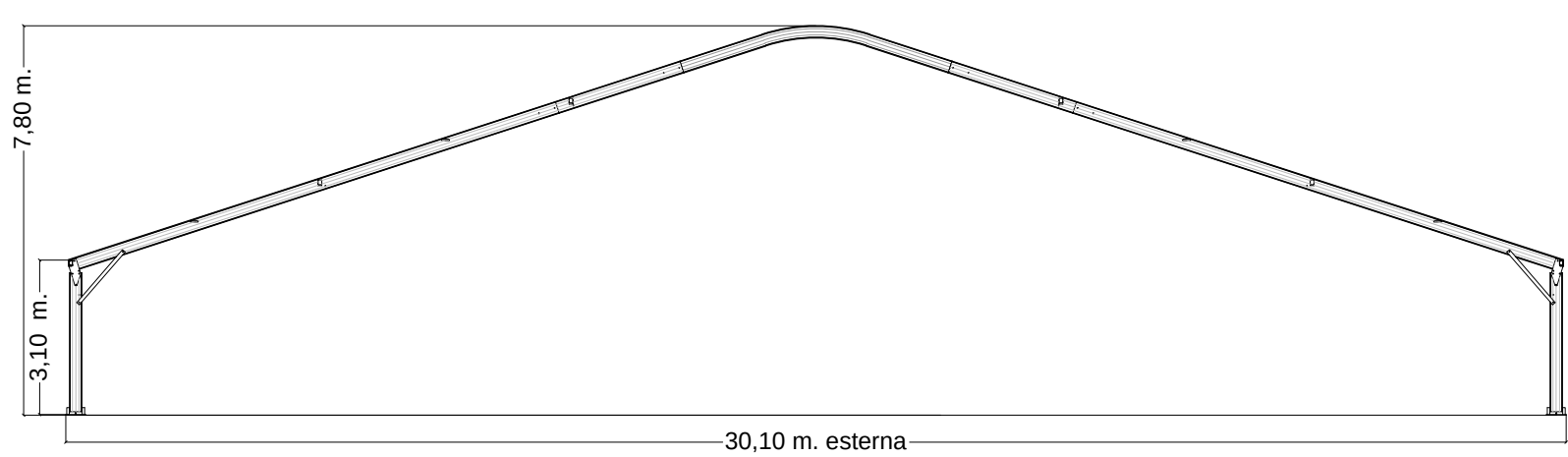
SEZIONE CENTRALE
