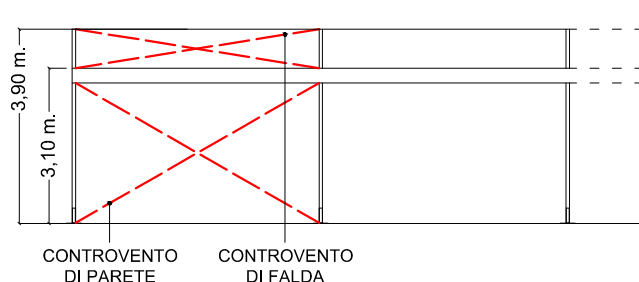
PROSPETTO LATERALE
