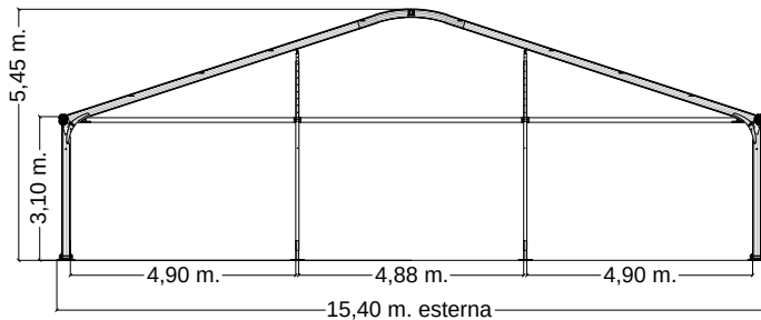
PROSPETTO FRONTALE
