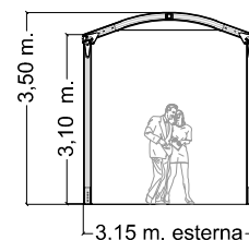
SEZIONE CENTRALE
