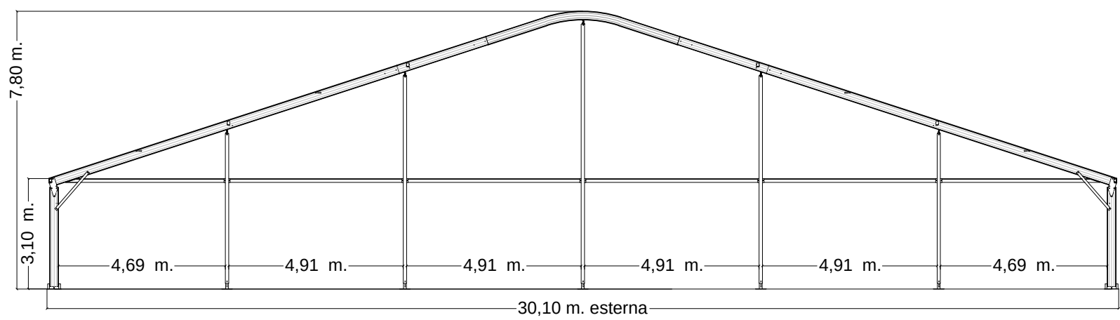
PROSPETTO FRONTALE
