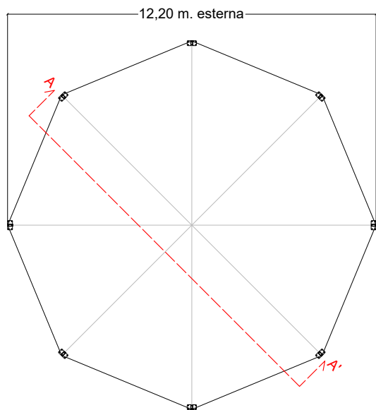
PLANIMETRIA
