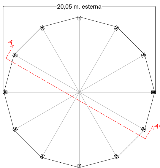
PLANIMETRIA
