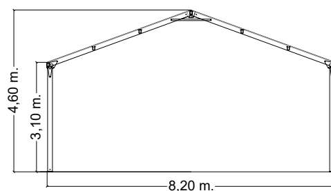
SEZIONE AA'
