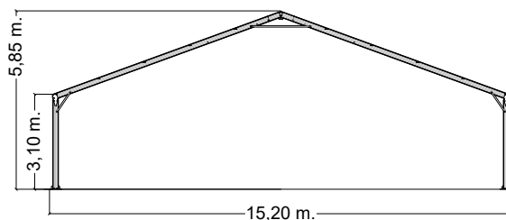
SEZIONE AA'
