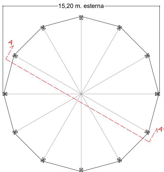
PLANIMETRIA
