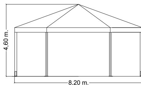
PROSPETTO FRONTALE
