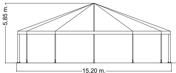
PROSPETTO FRONTALE
