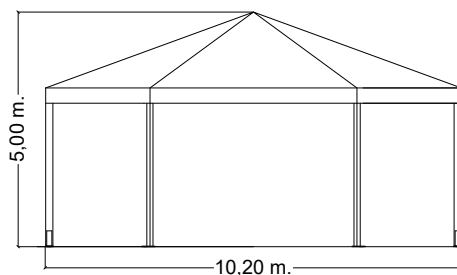
PROSPETTO FRONTALE
