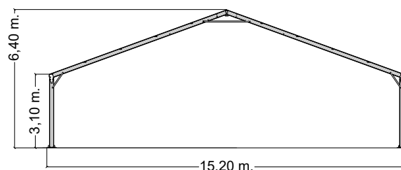
SEZIONE AA'
