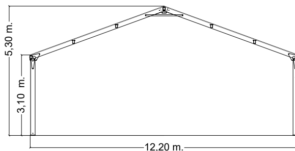
SEZIONE AA'
