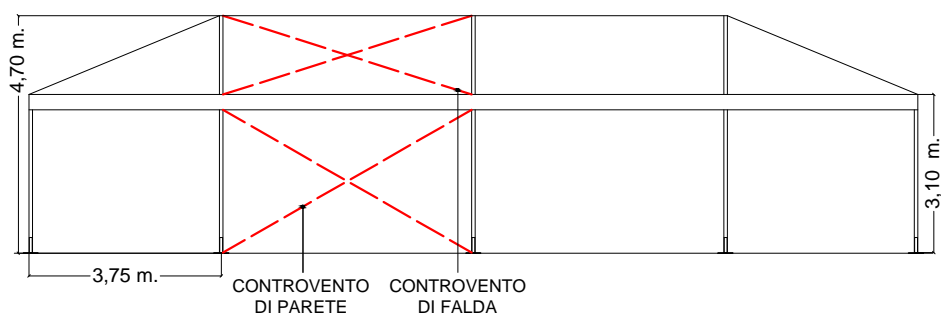
PROSPETTO LATERALE
