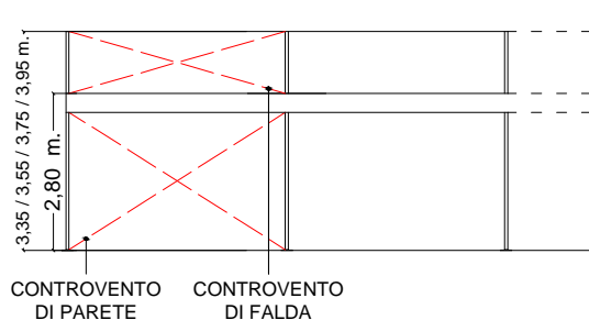
PROSPETTO LATERALE
