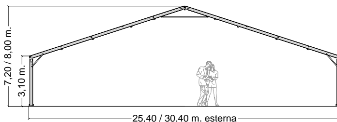
SEZIONE CENTRALE
