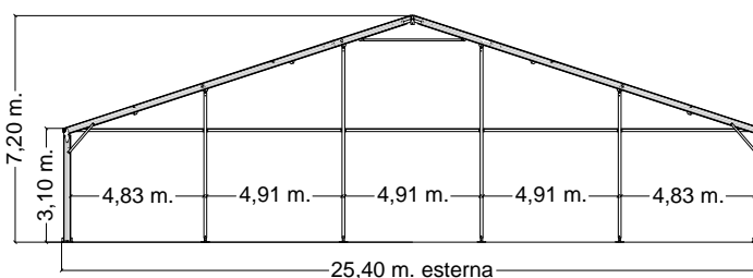
PROSPETTO FRONTALE PAD. 25 mt.
