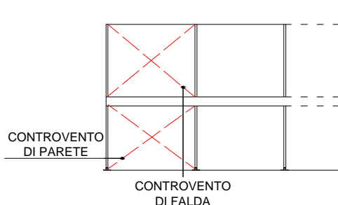
PROSPETTO LATERALE
