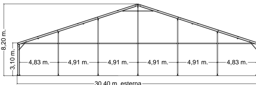
PROSPETTO FRONTALE PAD. 30 mt.
