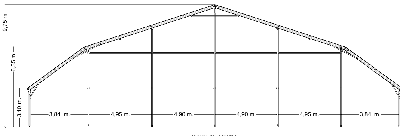
29,90 m. esterna PROSPETTO FRONTALE
