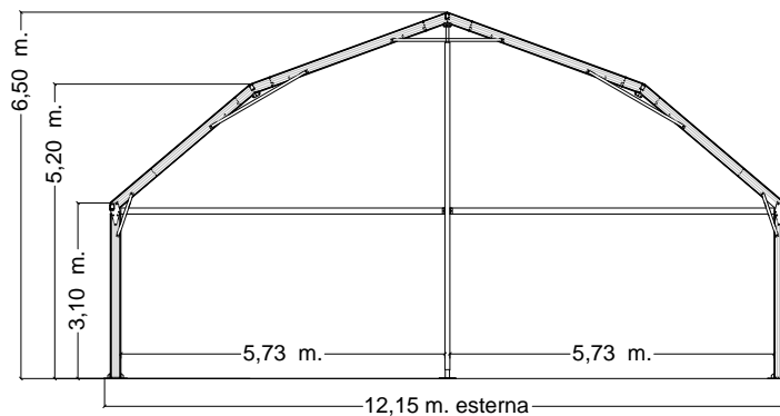
PROSPETTO FRONTALE
