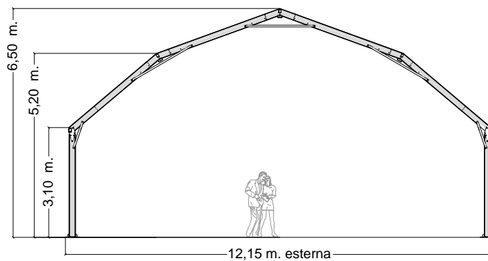
SEZIONE CENTRALE
