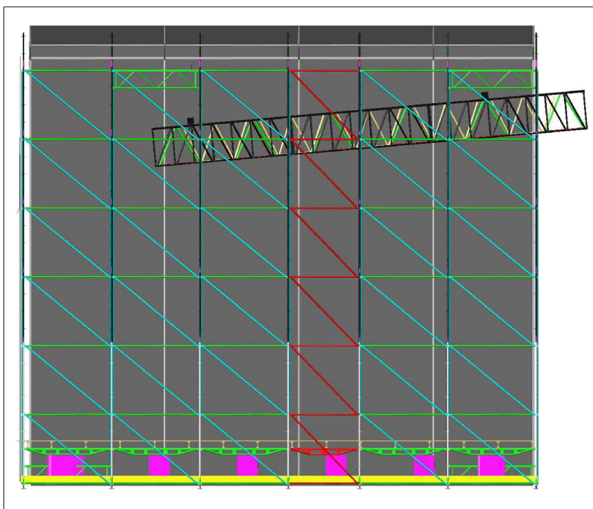
SEZIONE LATERALE
